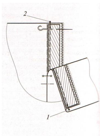
Притачивание второй стороны застежки-молнии (рис. 3)
